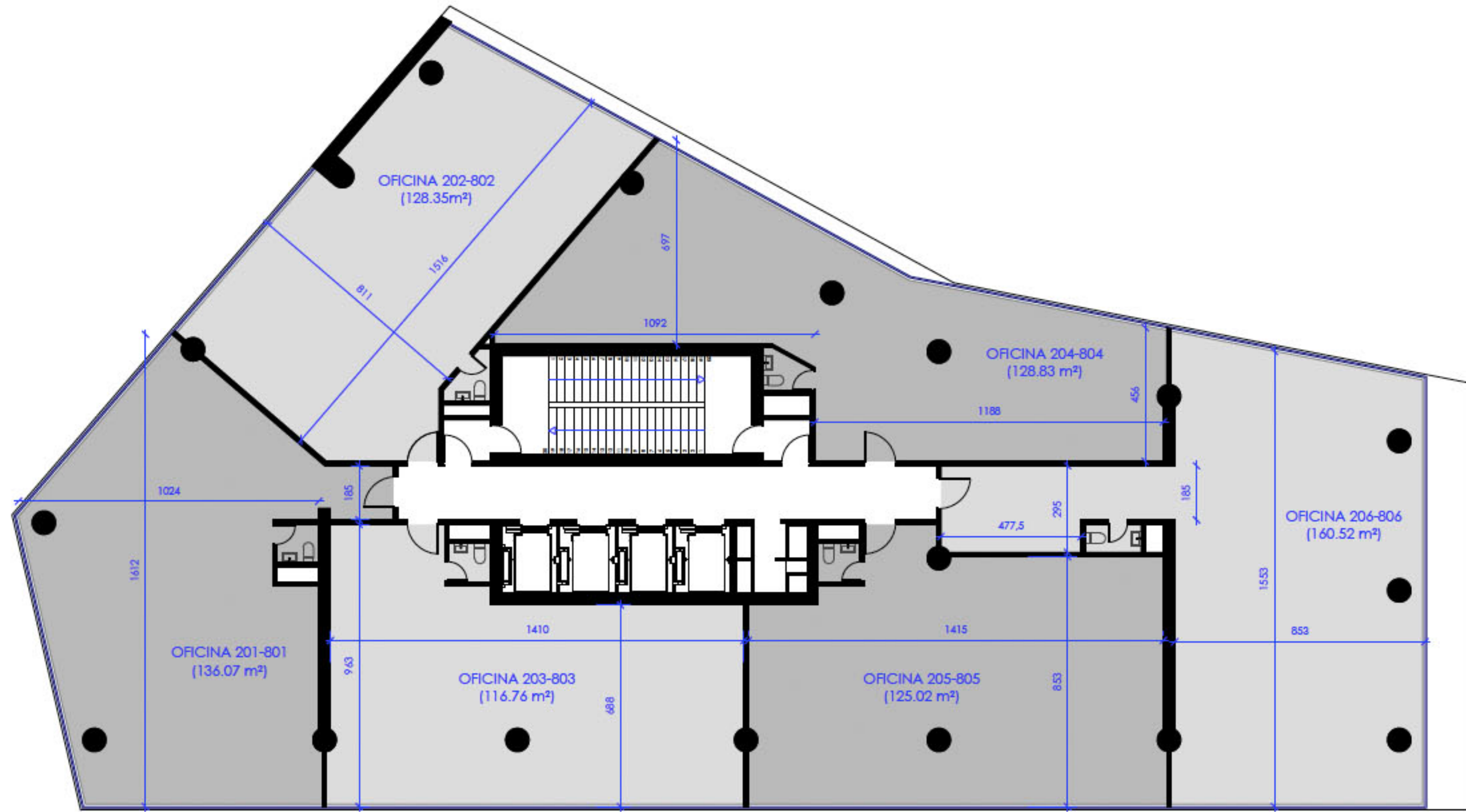
PLANTA NIVELES 2-8 ESCALA 1:100
